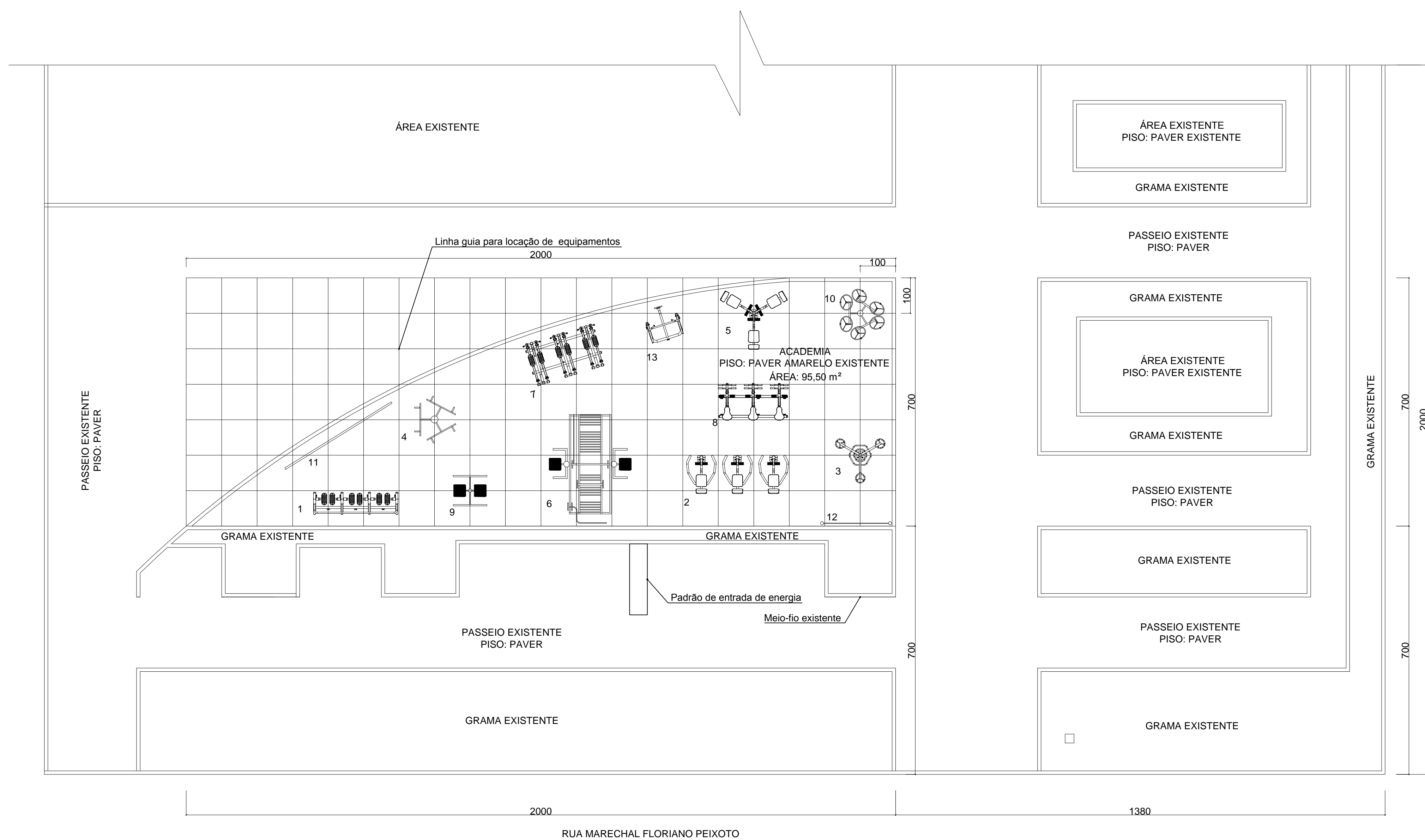
PLANTA BAIXA ACADEMIA AO AR LIVRE Escala 1/75
