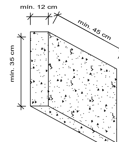
Dimensões Mínimas do Cordão de Pedra S/Escala
