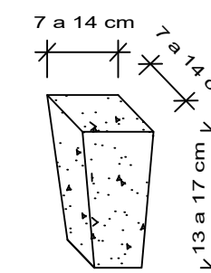
Dimensões das Pedra Irregulares S/Escala
