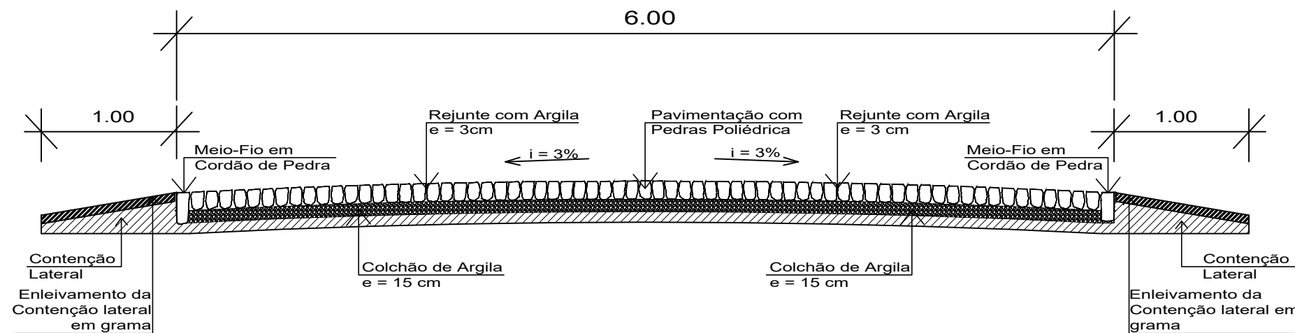
Seção transversal - Estrada Vicinal Extensão: 5.000m Área: 30.000m 2
