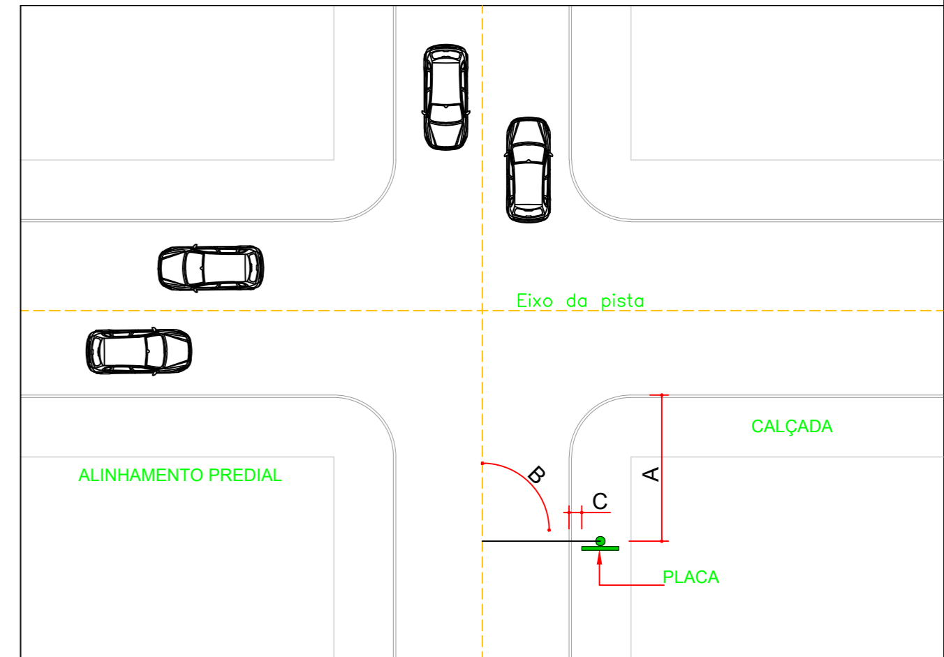
POSICIONAMENTO DA PLACA NA VIA
