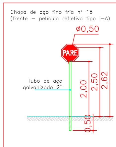
SINALIZAÇÃO VERTICAL - DETALHES SEM ESCALA (MEDIDAS EM METROS)
