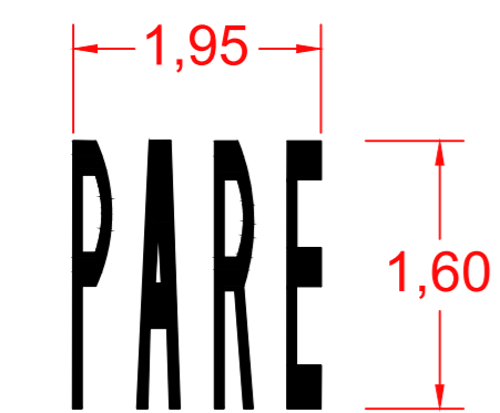
INSCRIÇÃO DE PAVIMENTO - DETALHES SEM ESCALA (MEDIDAS EM METROS)
