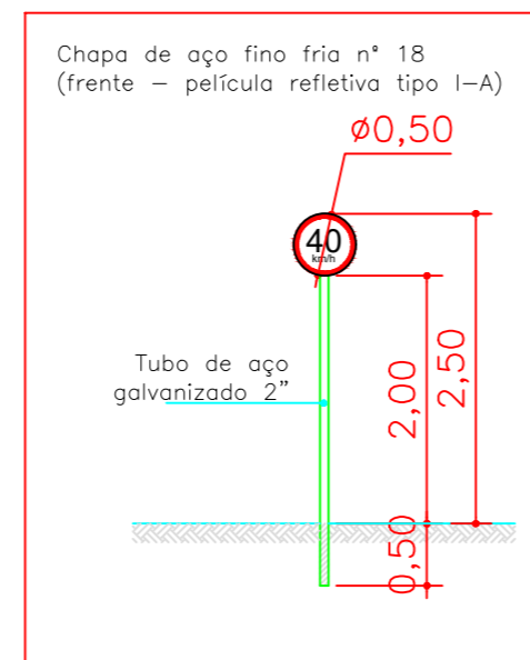
SINALIZAÇÃO VERTICAL - DETALHES SEM ESCALA (MEDIDAS EM METROS)
