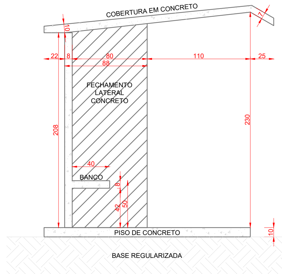
CORTE A-A
