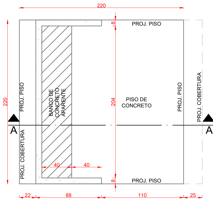
PLANTA BAIXA
