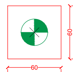
B1=B11=B13=B16=B19=B20 (1xC30)
