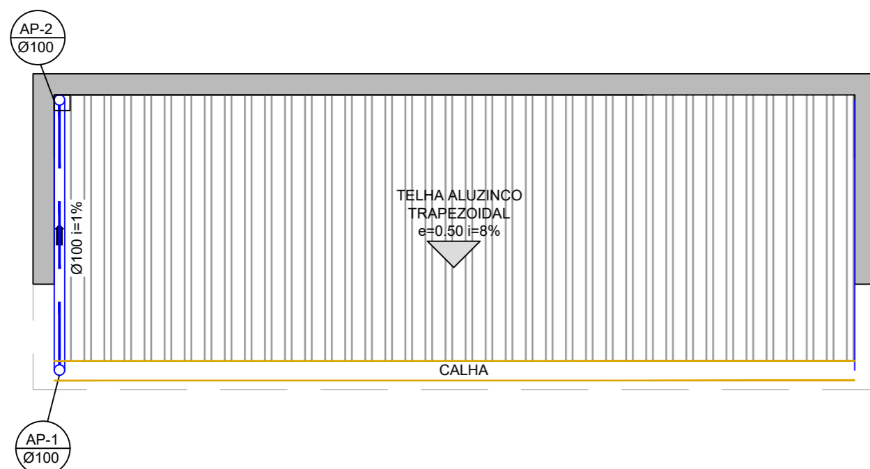
PLANTA COBERTURA ESC: 1/50
