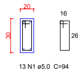
SEÇÃO A-A
